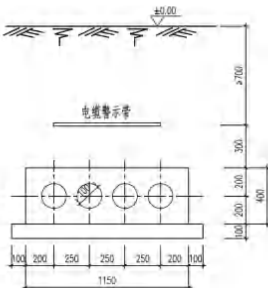
图 2.1-4 1×4 孔电缆排管断面图
