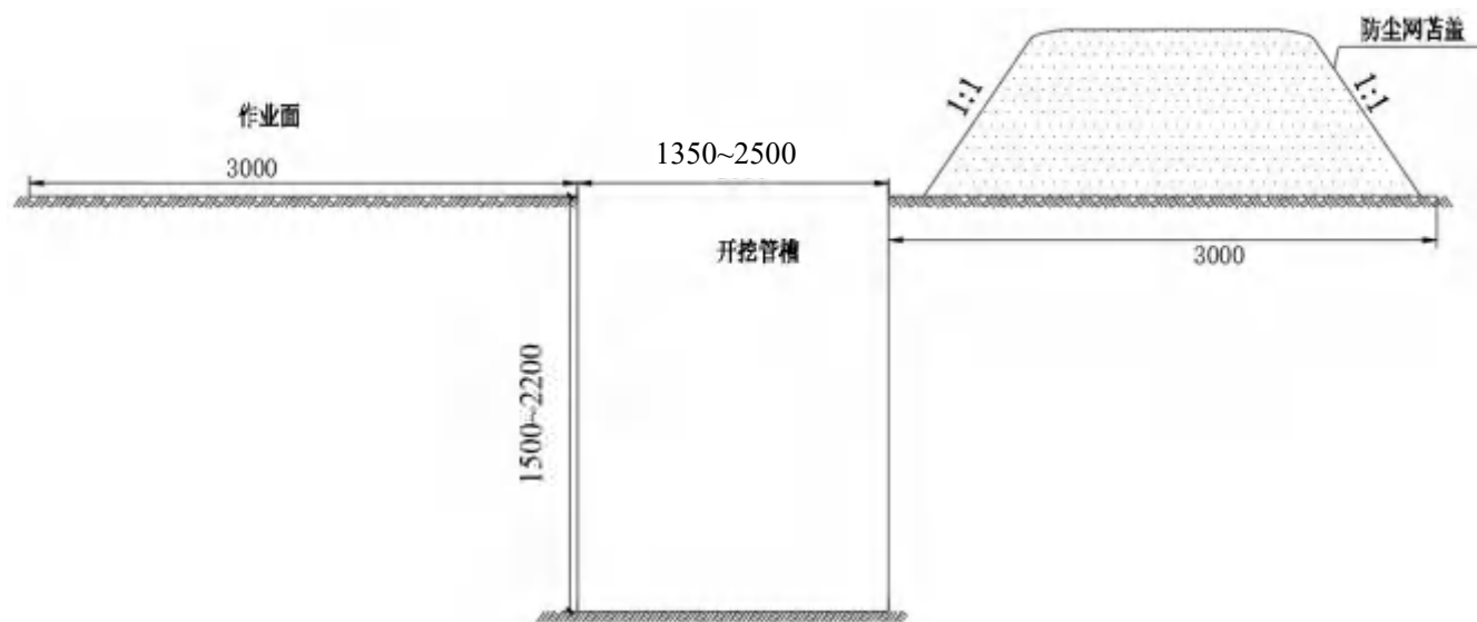
图 2.2-1 排管沟开挖作业面断面图
