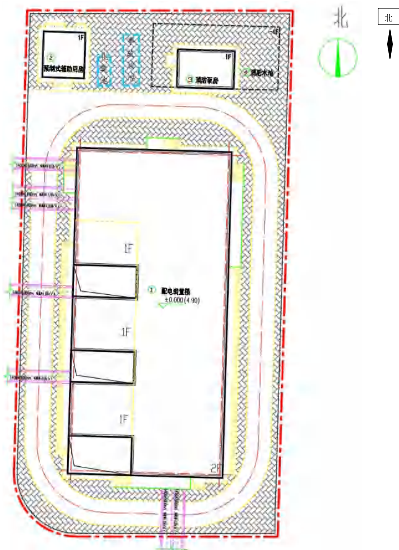
图 2.1-2 柳林变电站平面图
