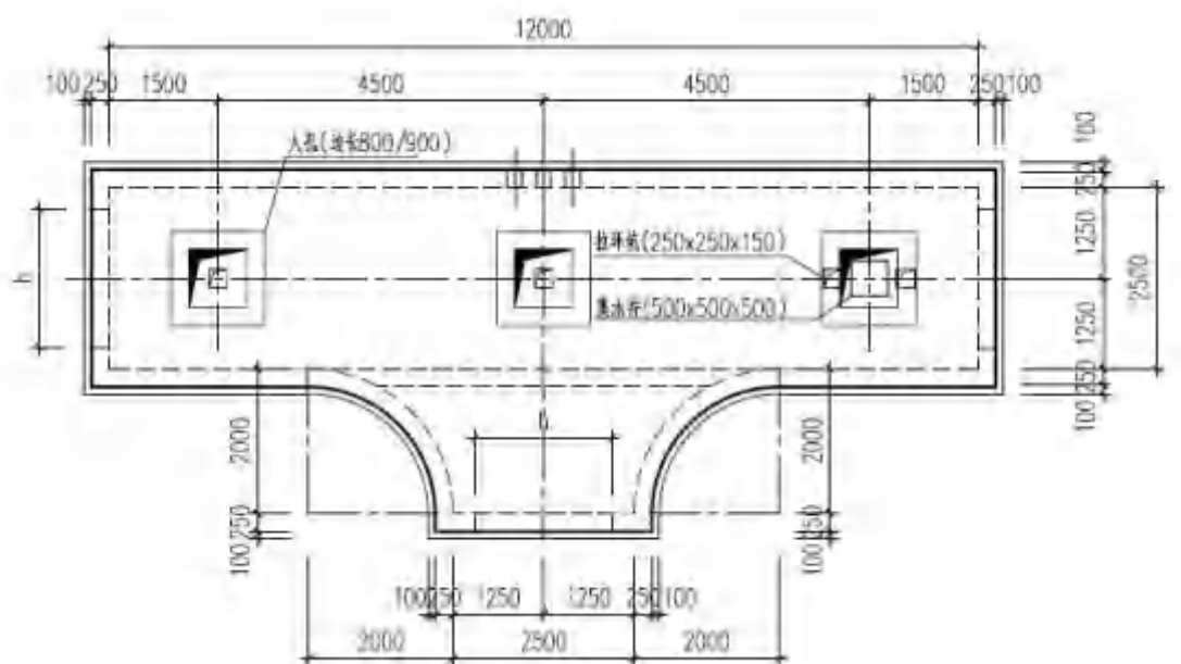
图 2.1-9 典型 T 型工井平面图
