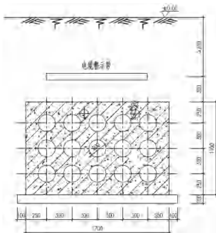
图 2.1-5 3×5 孔电缆排管断面图
