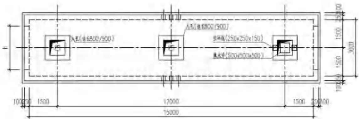
图 2.1-7 典型直线型工井平面图
