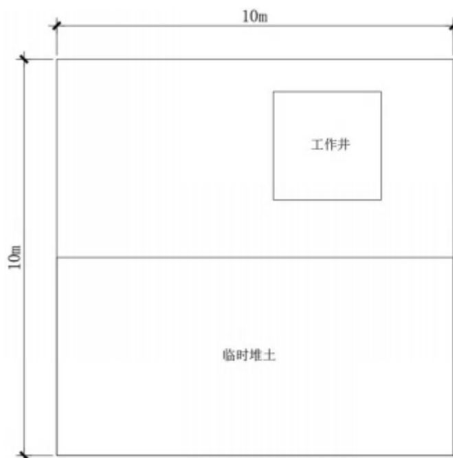
图 2.2-2 拉管施工布置图
