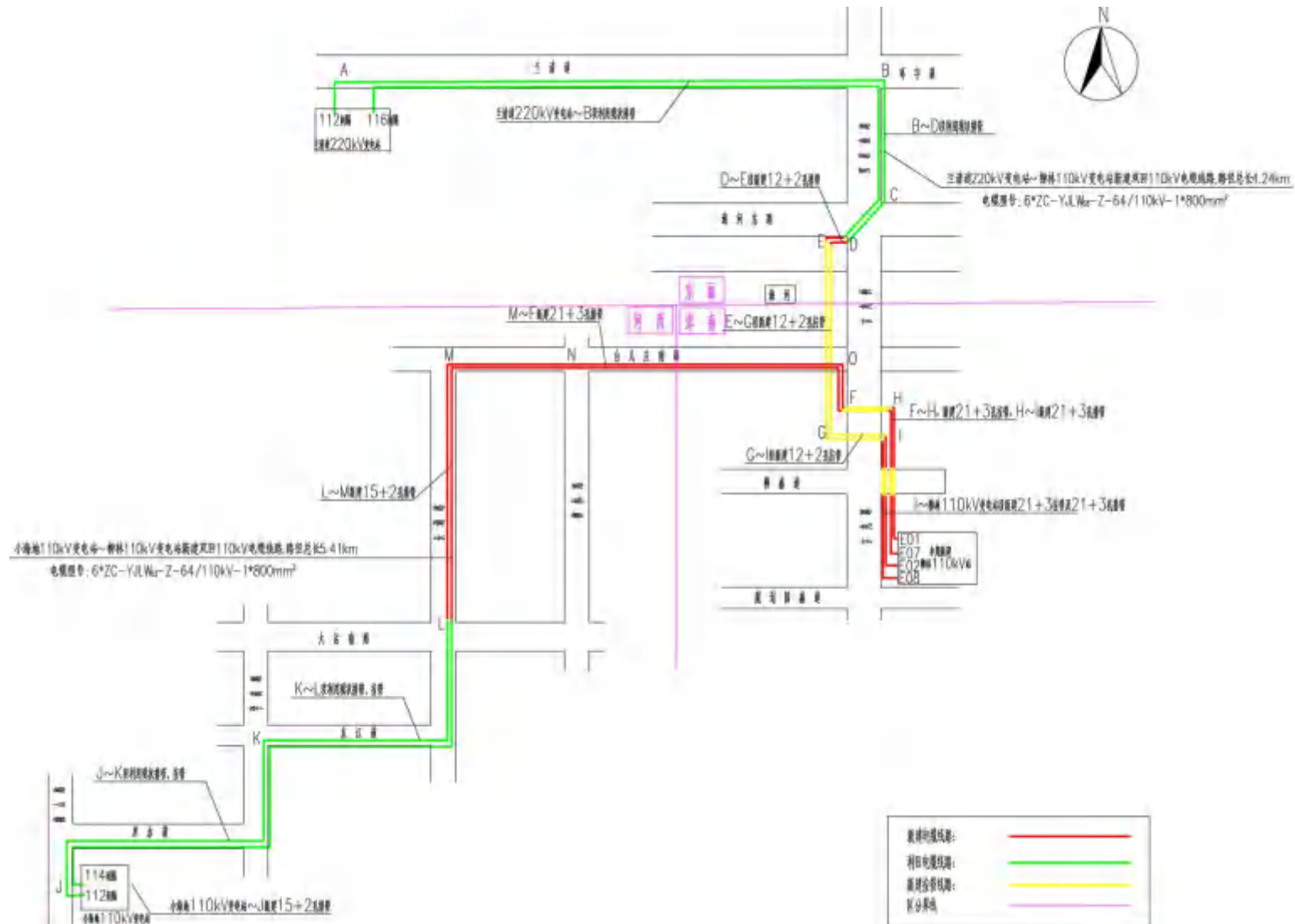
图 2.1-3 线路路径图
