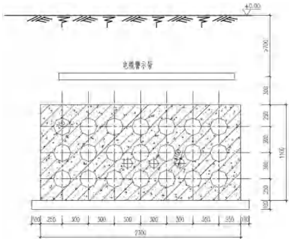
图 2.1-6 3×7 孔电缆排管断面图
