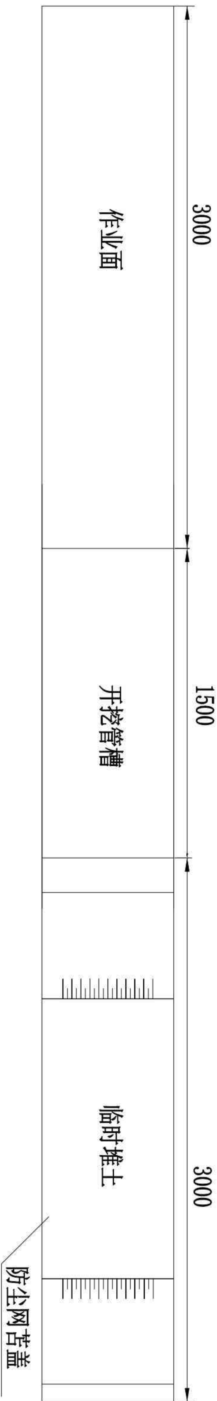
管沟开挖临时堆土防护平面布局图1:100
