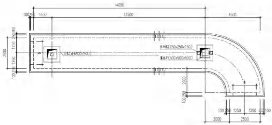
图 2.1-8 典型转角型工井平面图
